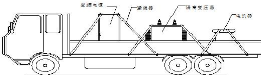
图 36 PY3520 型变频电源装置运输示意图
