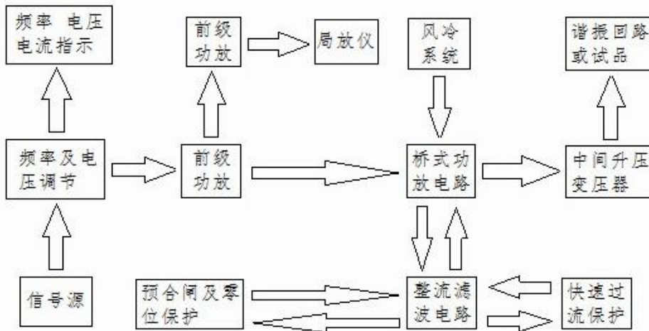
图1 PY3520型变频电源装置工作原理流程图
