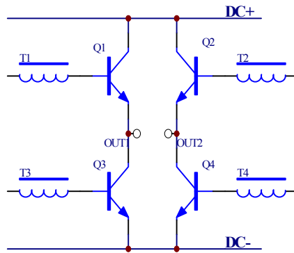
图 2 PY3520 型变频电源装置桥式放大电路原理图
