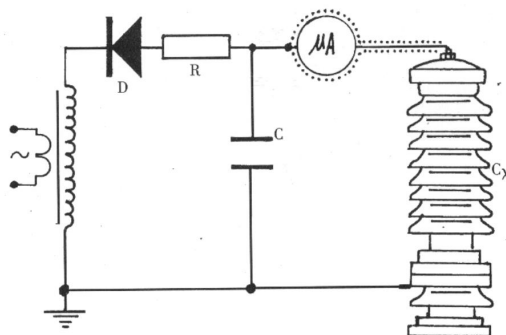
微安表接入试品 CX 高压侧接线图
