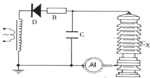
图 8a 微安表接入试品 C_X 底部的接线图
