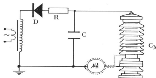
图 8b 排除试品 C_X 表面影响接线图
