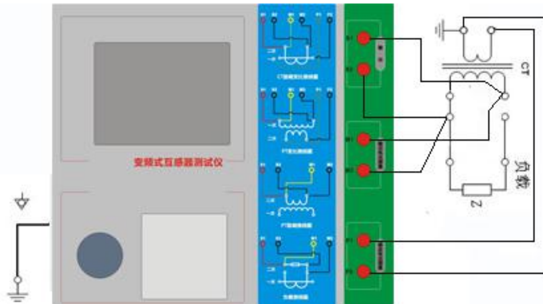
图 2.1 CT 直阻、励磁、变比试验接线方式
