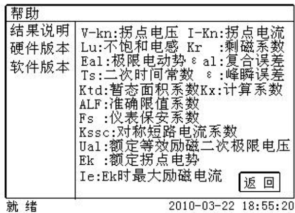
图 2.15 帮助界面
